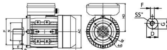
IMB14
