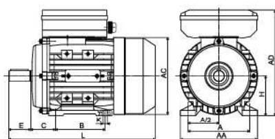
IMB3
